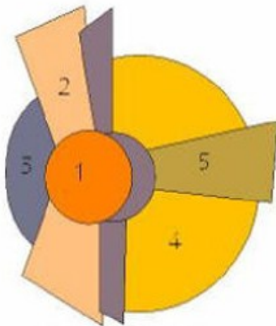
Sectormodel volgens Hoyt
