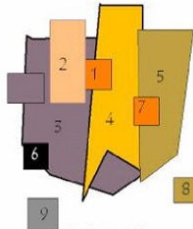
Meerkernenmodel volgens Harris&Ullman
